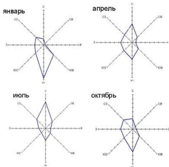
Рисунок 1 – Розы ветров
