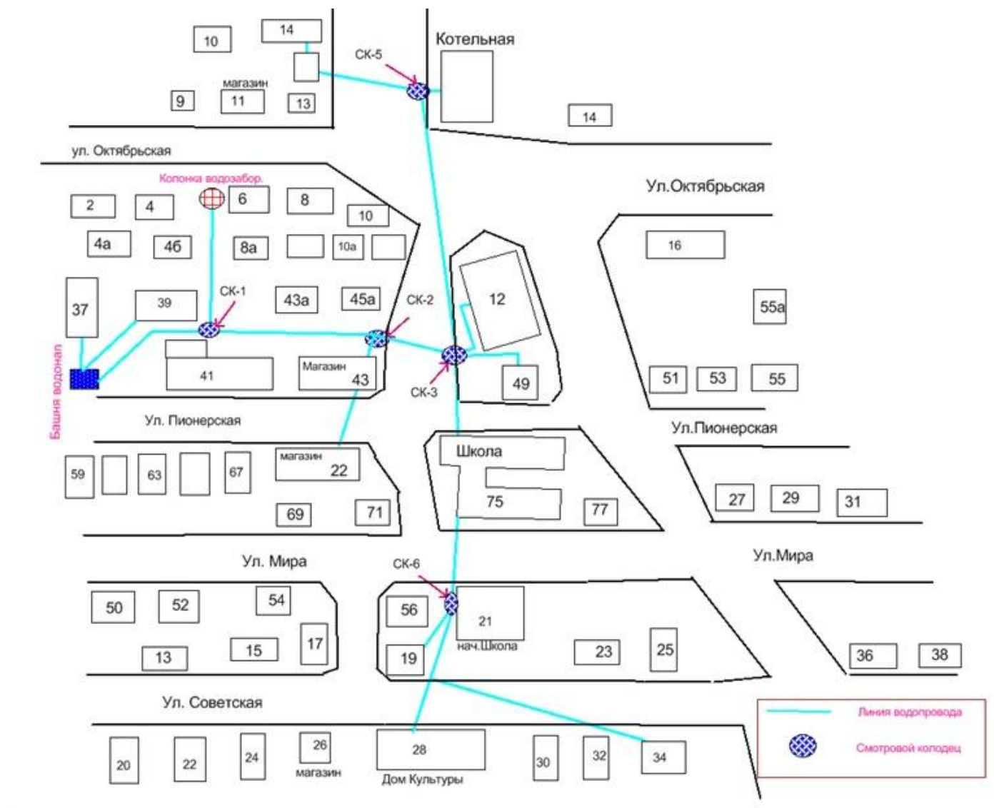
Схема существующего размещения объектов централизованной системы водоснабжения в д. Кушкопала МО «Кушкопальское»
